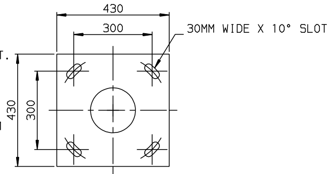
FLANGE PLATE OPTION SCALE: 1:10
